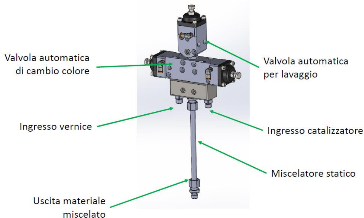
Testa di miscelazione 250 bar, 1/4" Gas fietti
